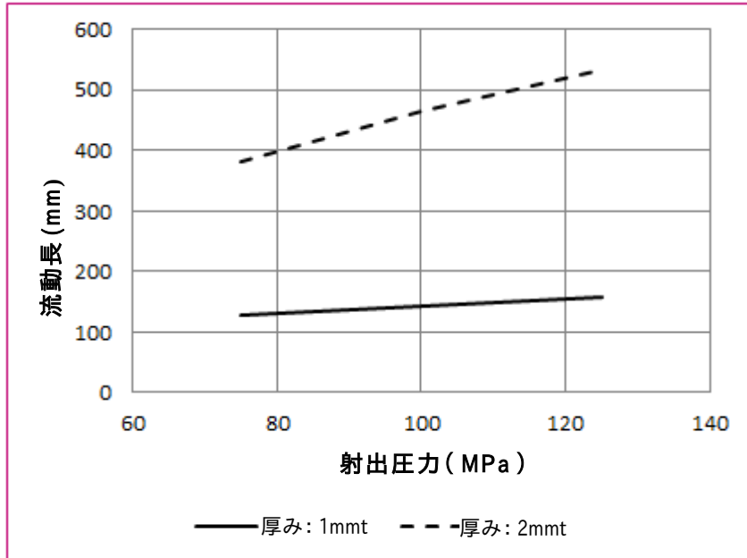
図3-1 ジュラファイド® PPS 6150T73の棒流動長
