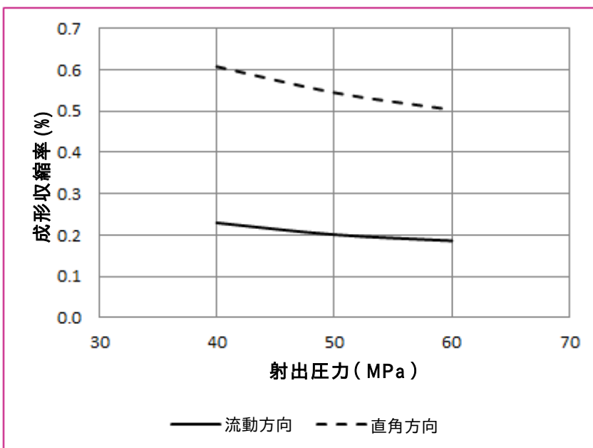
図3-2 ジュラファイド® PPS 6150T73の成形収縮率
