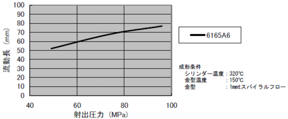
(図 3-1) 流動長(1mmt)
