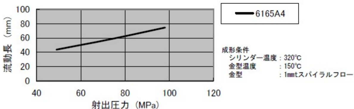
(図 3-1) 流動長(1mmt)
