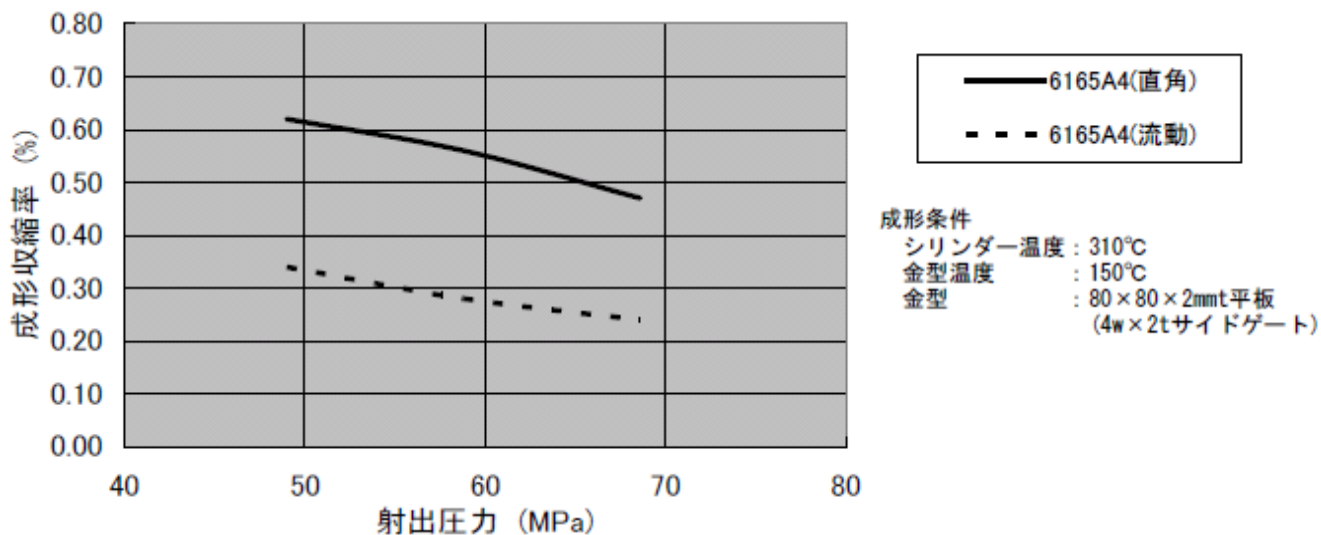
(図 3-2) 成形収縮率(80□×2mmt)
