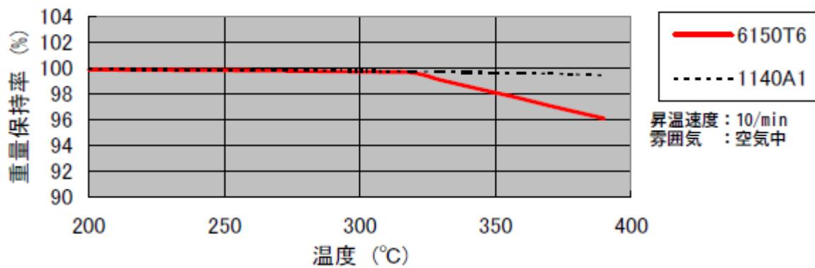
(図 4-1) 熱重量曲線
