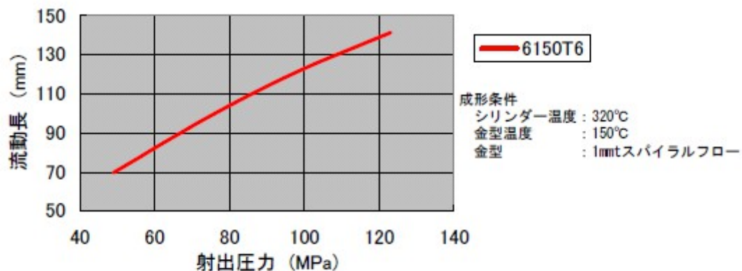
(図 5-1) 流動長(1mmt)
