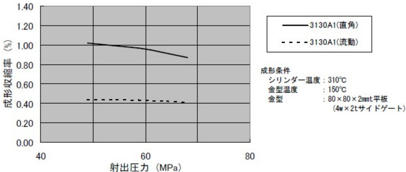
(図 3-2) 成形収縮率(80□×2mmt)
