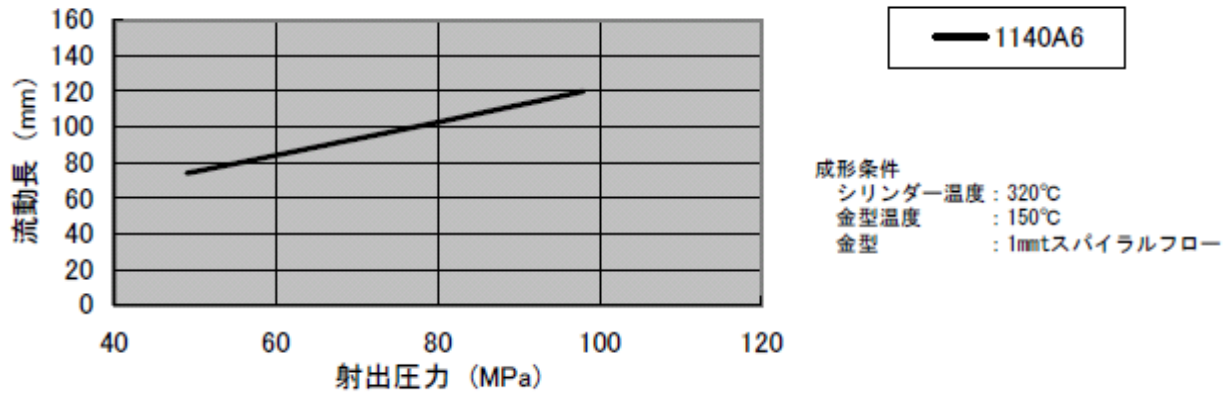
(図 3-1) 流動長(1mmt)
