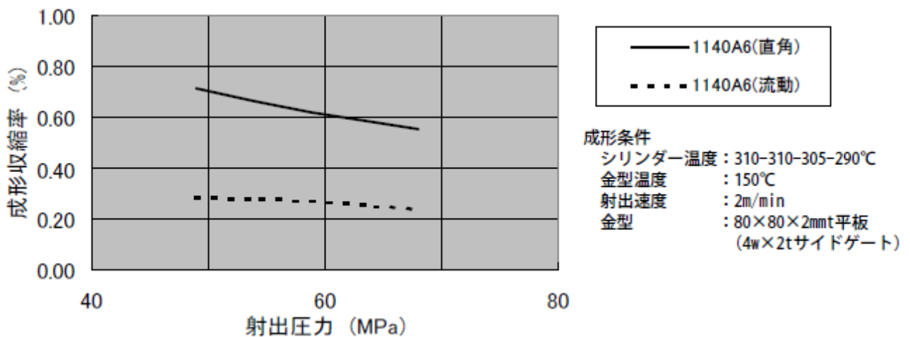
(図 3-2) 成形収縮率(80□×2mmt)
