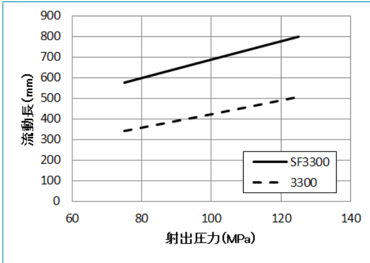
図3-1 棒流動長(2mm)
