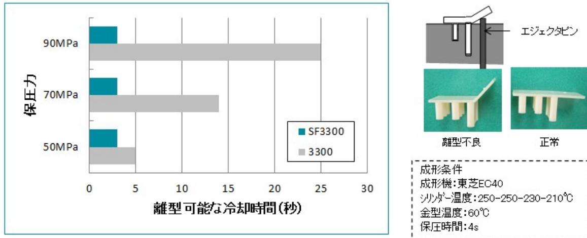
図2-1 SF3300と3300の離型性能比較
