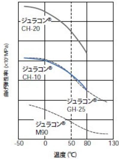
図2-1 曲げ弾性率の温度依存性
