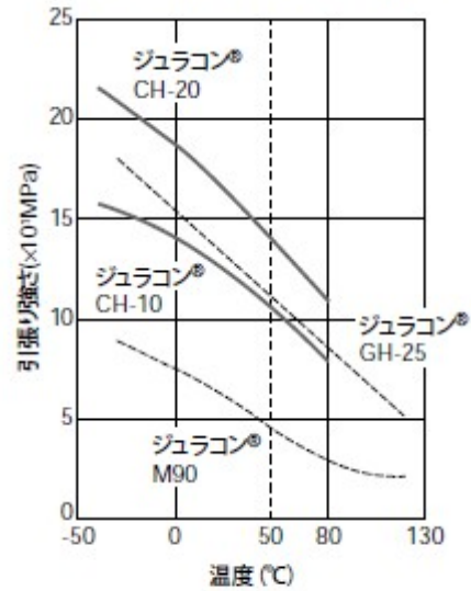
図2-2 引張り強さの温度依存性
