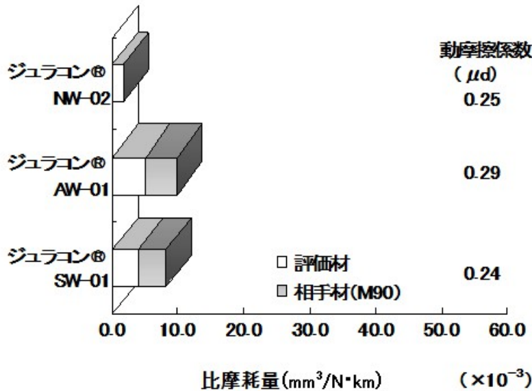
図 1-4 中負荷 低温 (-10℃) 摩擦摩耗特性(鈴木式摺動)
