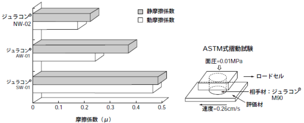
図 1-1 軽負荷 摩擦係数 (ASTM式摺動)
