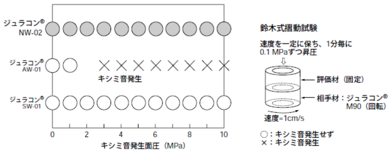
図 2-1 キシミ音特性
