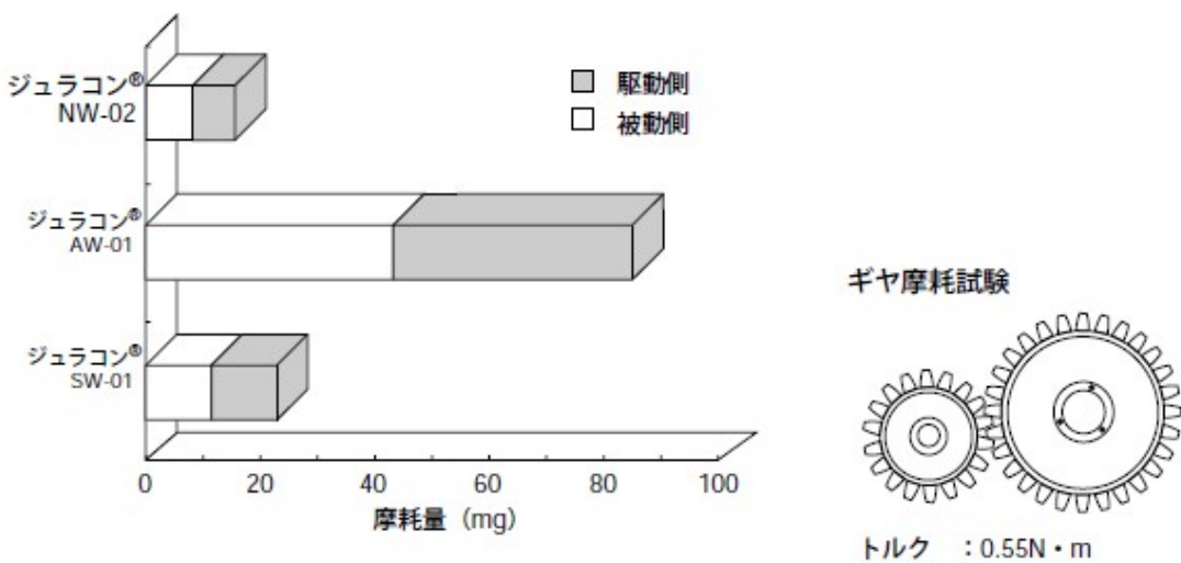
図 1-7 高負荷 ギヤ摩耗特性(同材)
