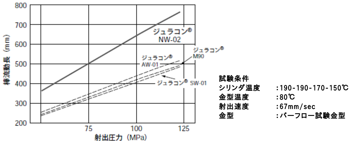
図 3-1 棒流動長(2mnt)
