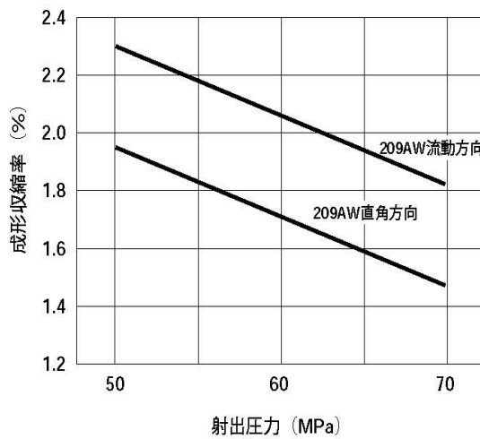
図5 成形収縮率 (120 \square \times 2mm t )
