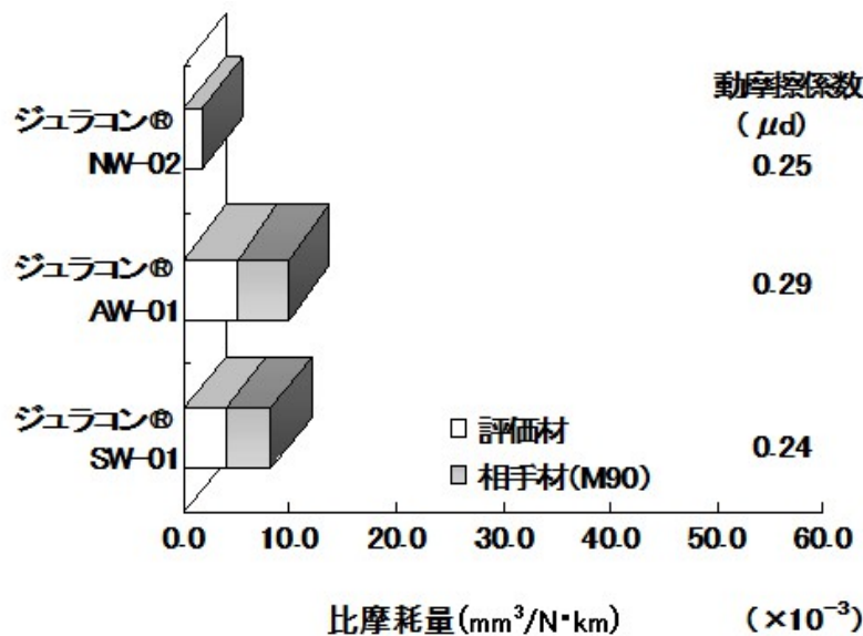
図 1-5 高負荷 摩擦摩耗特性 (往復摺動)
