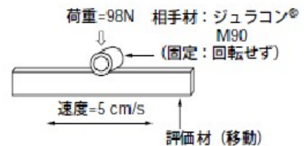
往復摺動試験
