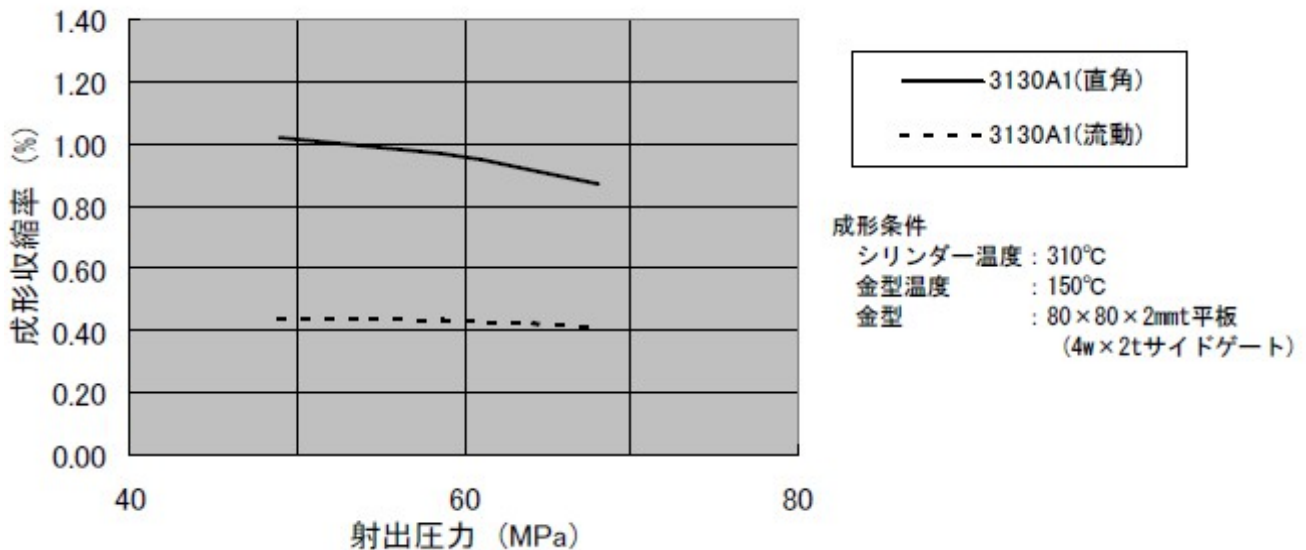
図 3-2 成形収縮率(80□×2mmt)
