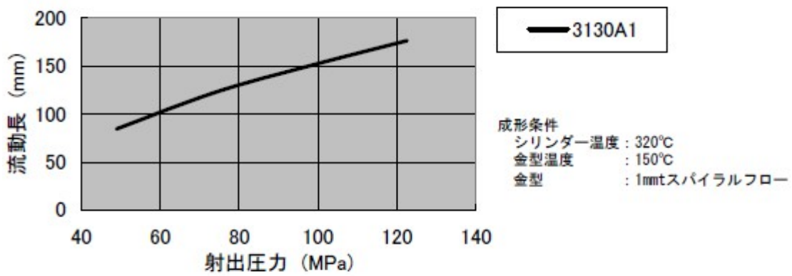
図 3-1 流動長(1mmt)
