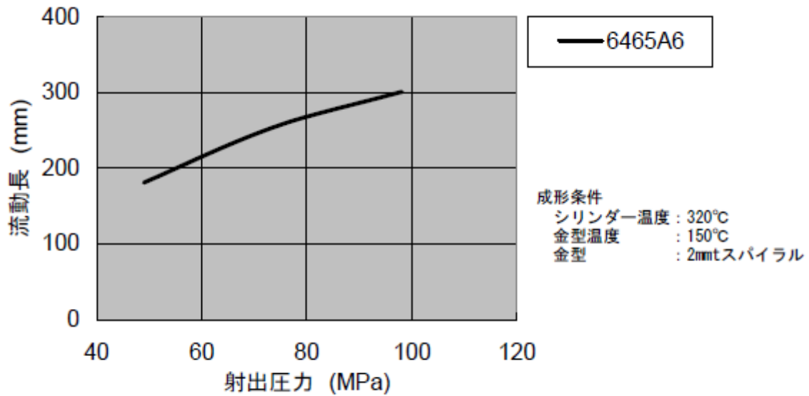
図 3-1 流動長(2mmt)
