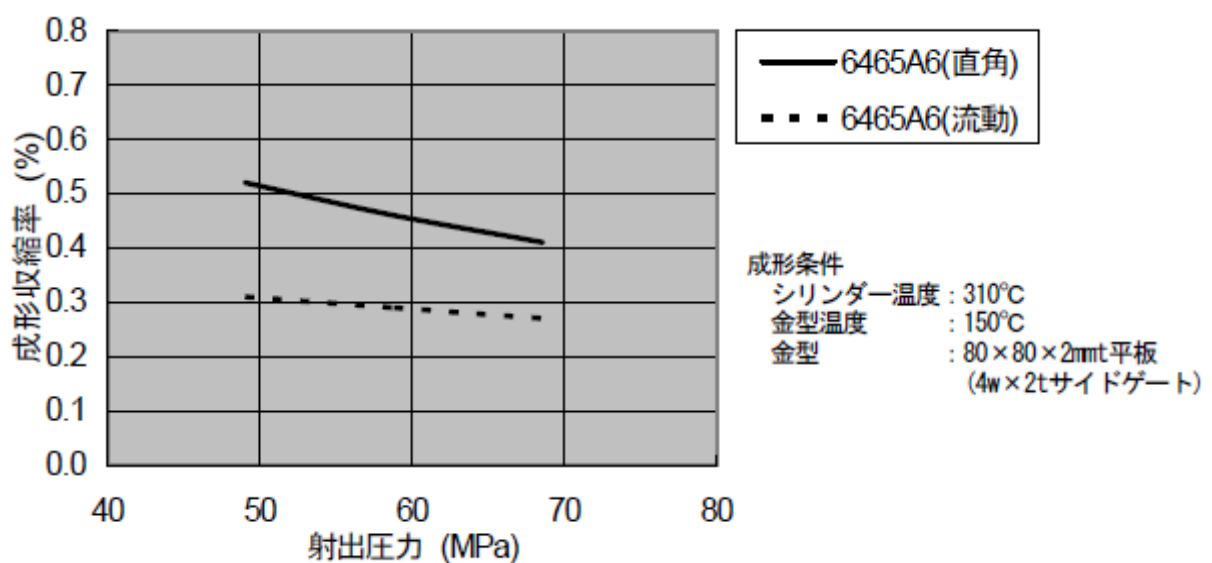
図 3-2 成形収縮率(80□×2mmt)
