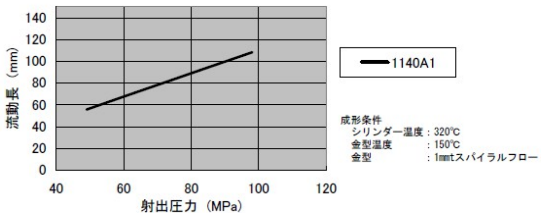
図 5-1 流動長(1mmt)
