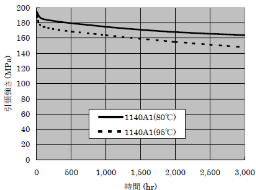
図 3-1 耐熱水性
