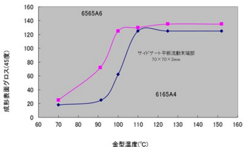
(図 3-5) 成形表面性と金型温度の関係
