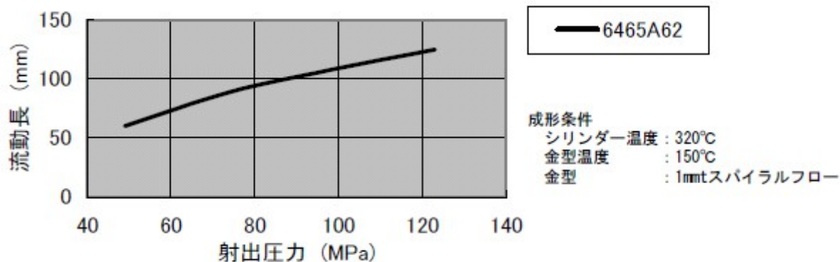
図 3-1 流動長(1mmt)
