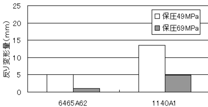
図 4-1 平板の反り変形量(120mm□×2mmt)
