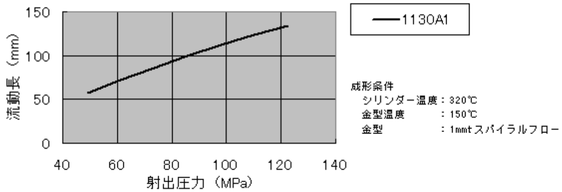
図 3-1 流動長(1mmt)
