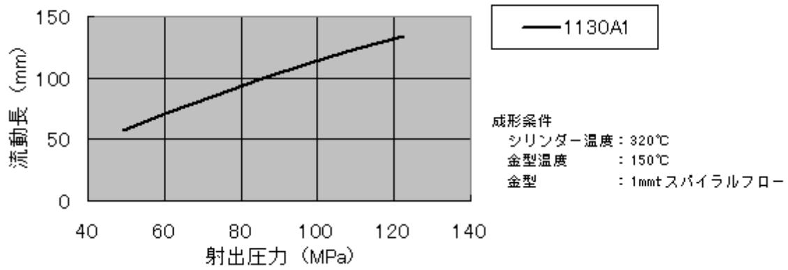
(図 3-1) 流動長(1mmt)
