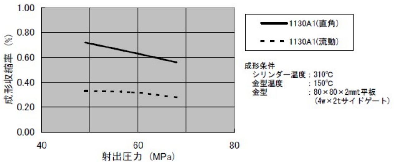
(図 3-2) 成形収縮率(80□×2mmt)
