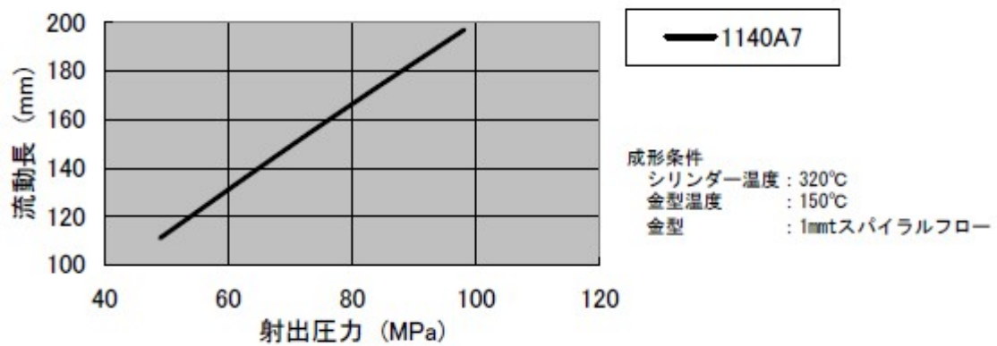
(図 5-1) 流動長(1mmt)
