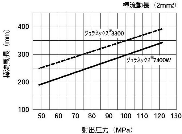
図4-1 ジュラネックス®7400Wの流動性
