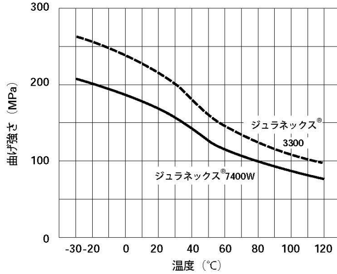
図2-1 曲げ強さの温度依存性
