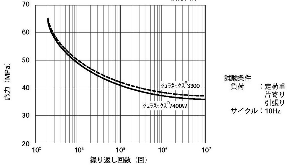
図3-1 ジュラネックス®7400Wの疲労曲線 疲労曲線
