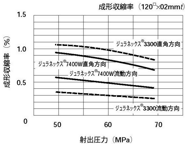
図4-2 ジュラネックス®7400Wの成形収縮率
