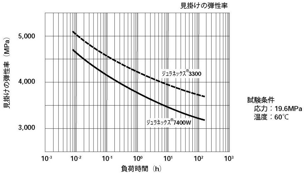
図3-2 ジュラネックス®7400Wの曲げクリープ特性
