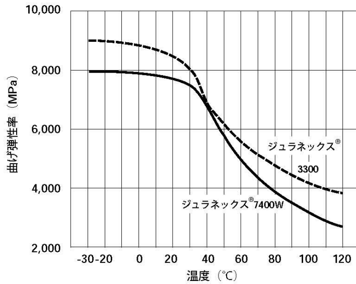
図2-2 曲げ弾性率の温度依存性
