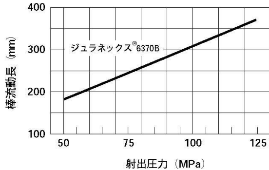
図2-1. 棒流動長 (2mm t )
