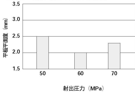
図2-3. 平板平面度 (120 \square ×2mm t )
