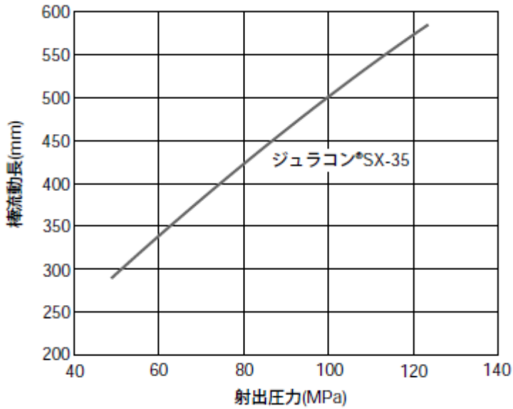
図1-1. 棒流動長(2mmt)
