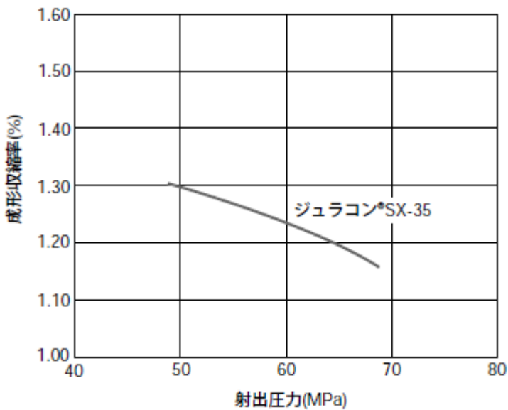
図1-2. 成形収縮率(2mmt)
