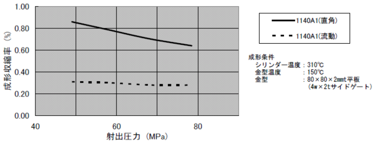
(図 5-2) 成形収縮率(80口×2mmt)
