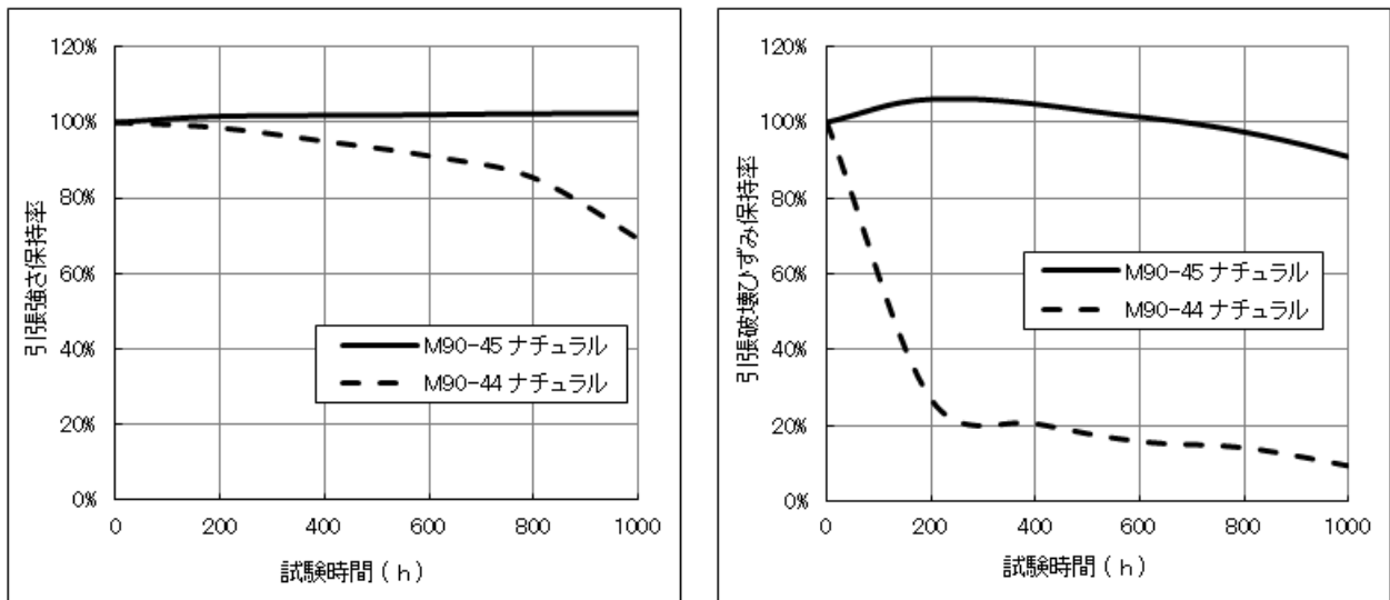
サンシャインカーボンアーク灯式耐候性試験 JIS D0205 WAN-1S ブラックパネル温度 63°C、水噴射あり
