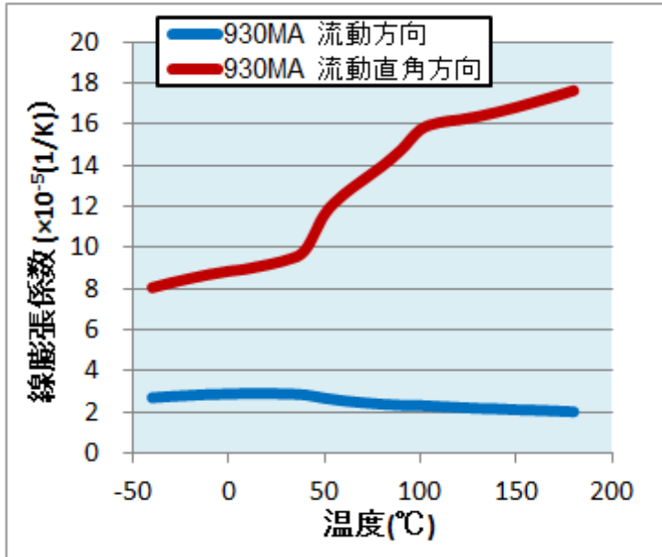
圖4-1. 線膨脹係數
