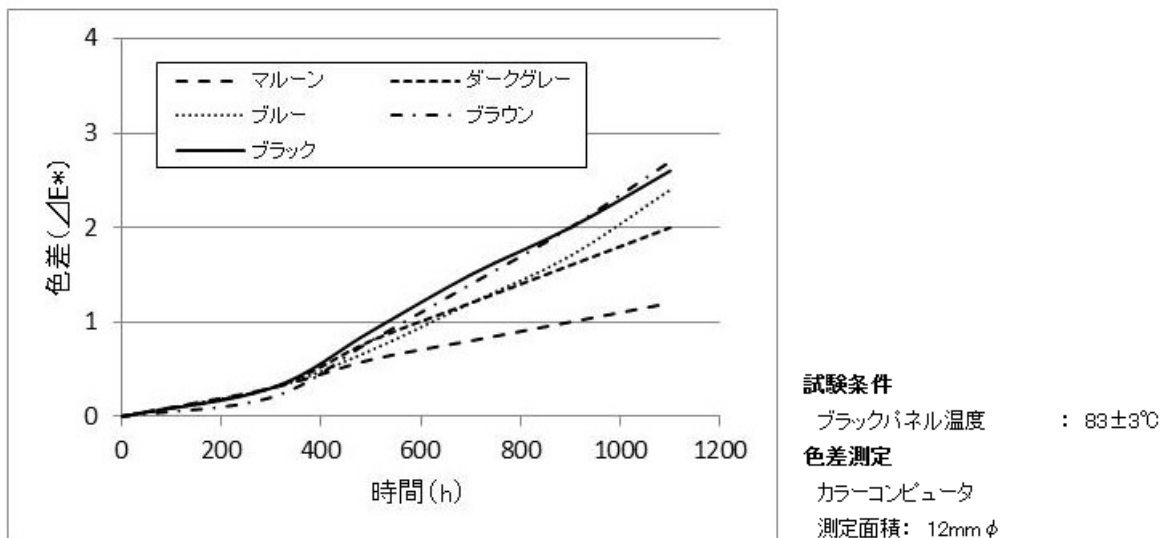
図 2-2 LU-02の紫外線フェードメーターにおける色差(ΔE*)
