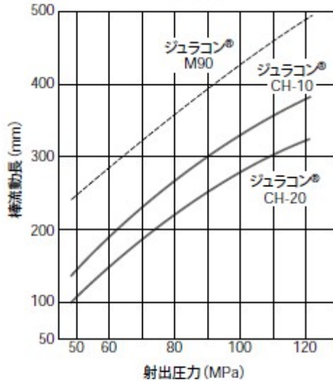
図5-1 棒流動長 (2mmt)
