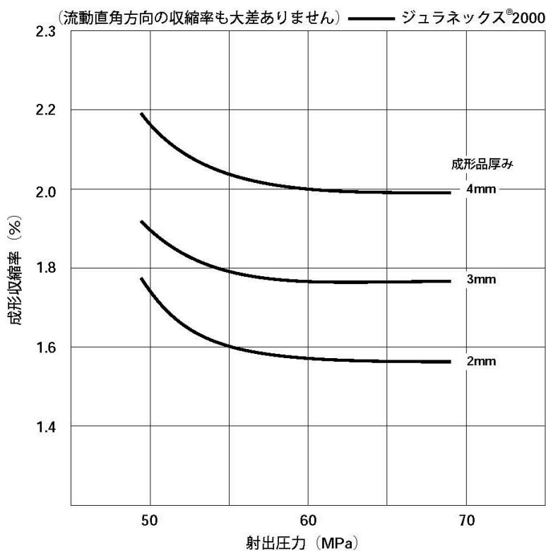
図2-2 ジュラネックス®2000の流動方向の成形収縮率 (%)
