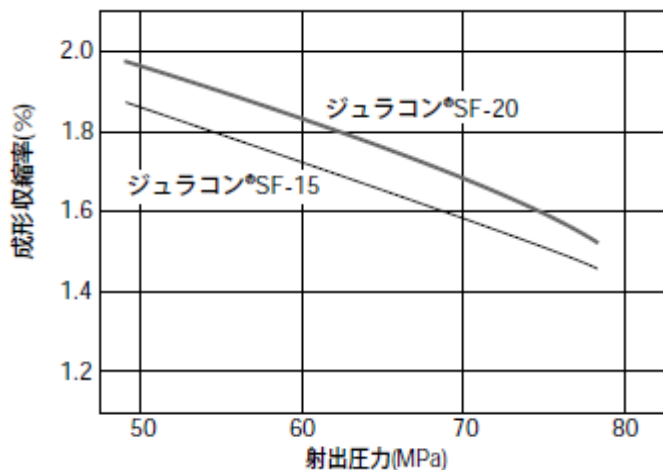
図1-3 成形収縮率(120口×2mmt)
