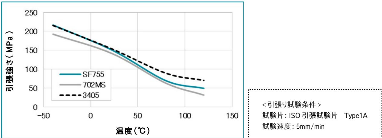
図6-1 SF755と従来グレードの引張強さ温度依存性比較
