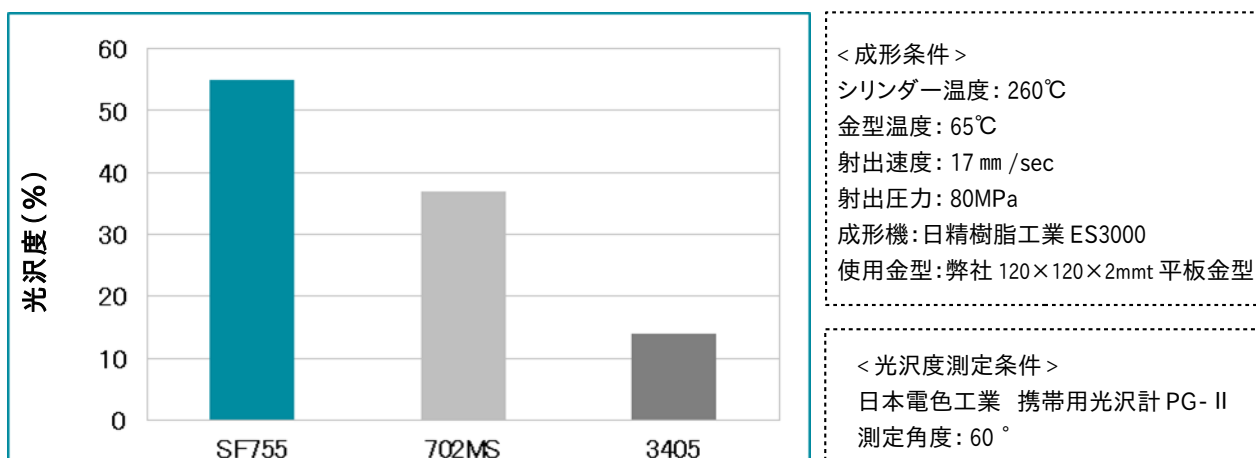
図4-1 SF755と従来グレードの光沢度比較
