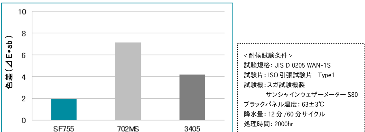
図7-1 SF755と従来グレードの耐候性比較
