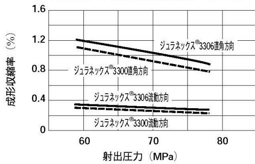
ジュラネックス®3306の成形収縮率 (2mmt)
