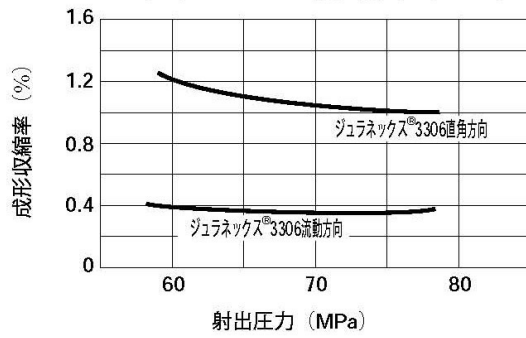
ジュラネックス®3306の成形収縮率 (3mmt)
