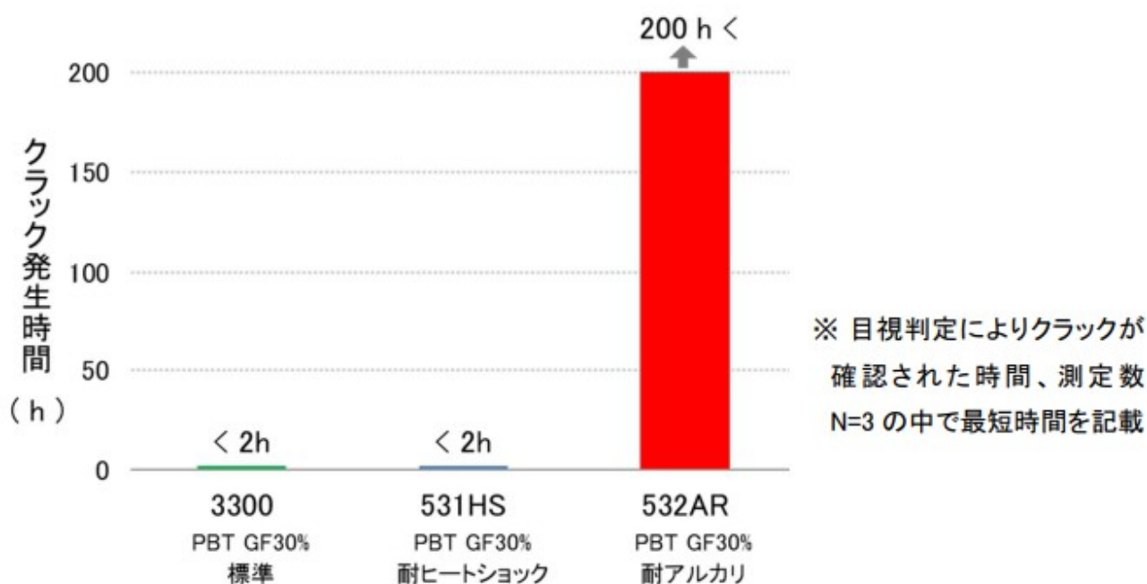
図2-2 アルカリ環境下におけるストレスクラックの発生時間
