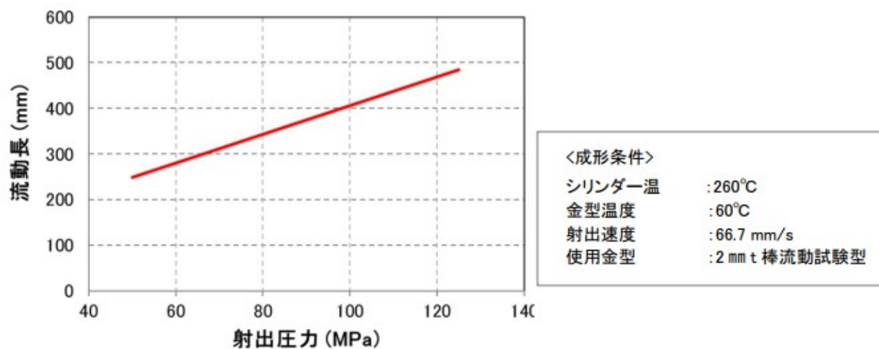
図5-1 ジュラネックス® PBT 532AR 流動性
