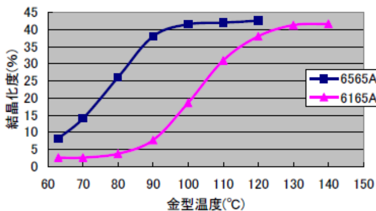
図 3-3 結晶化度と金型温度の関係
