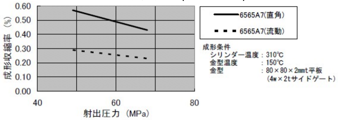
図 3-2 成形収縮率(80口×2mmt)
