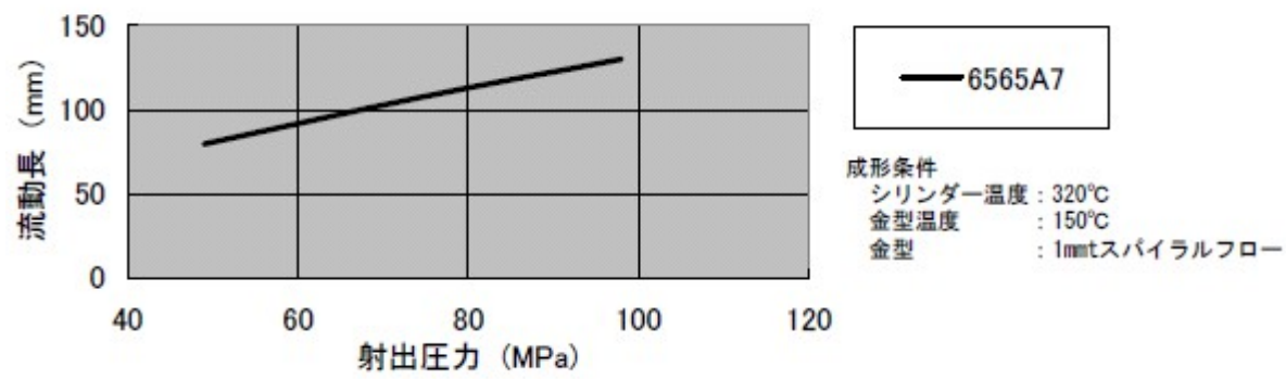
図 3-1 流動長(1mmt)
