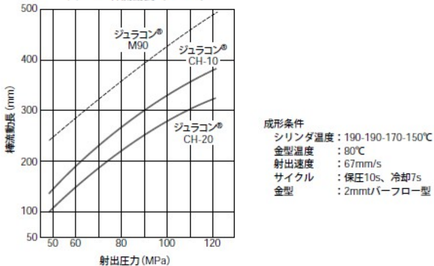
図5-1 棒流動長 (2mm)
