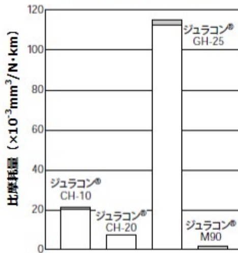
図4-1 対金属での比摩耗量
