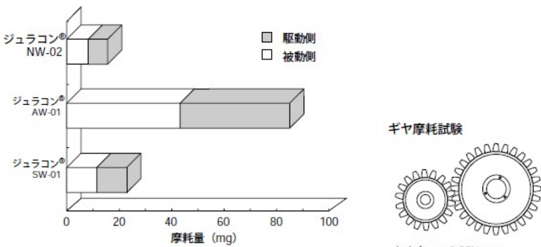
図 1-7 高負荷 ギヤ摩耗特性(同材)
