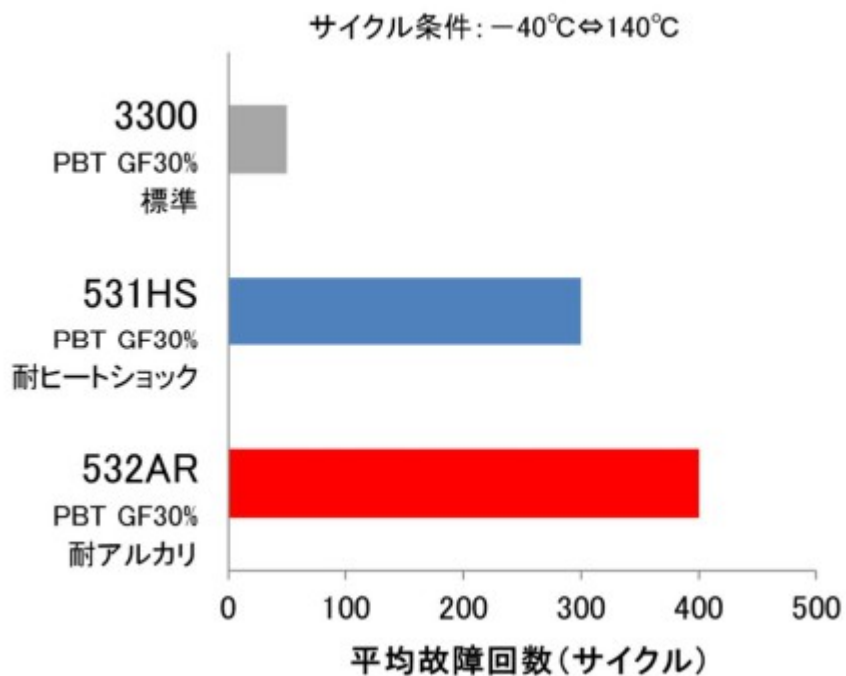
図3-1 ジュラネックス® PBT 532AR と 531HS との耐ヒートショック性
