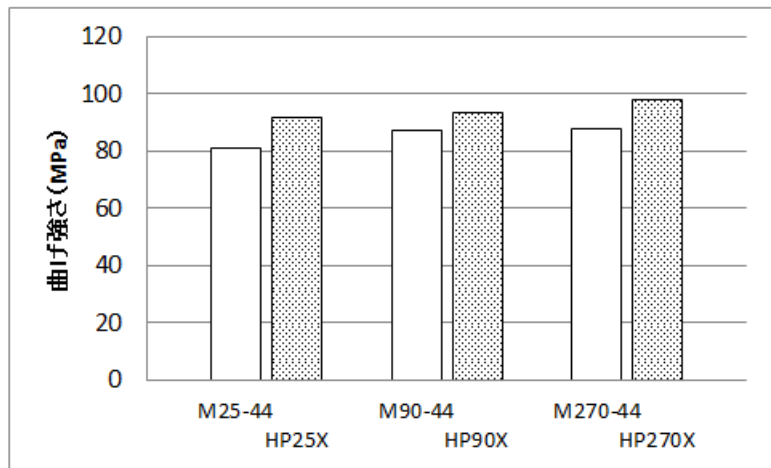
図 1-3 HP-Xシリーズと一般グレードの曲げ強さの比較 (ISO 178, 23℃)
