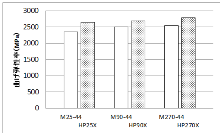
図 1-4 HP-Xシリーズと一般グレードの曲げ弾性率の比較 (ISO 178, 23℃)
