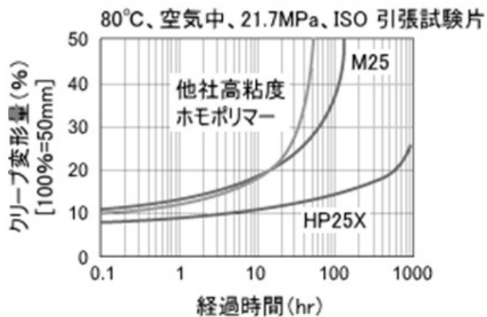
図 2-4 クリープ変形特性(引張クリープ試験)
