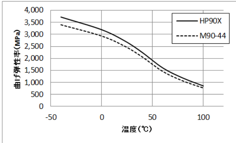
図 1-5 曲げ弾性率の温度依存性 (ISO 178)
