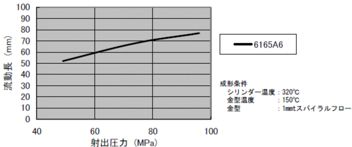
図 3-1 流動長(1mmt)
