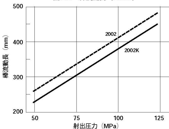
図2-2 棒流動長 (2mm \phi )
