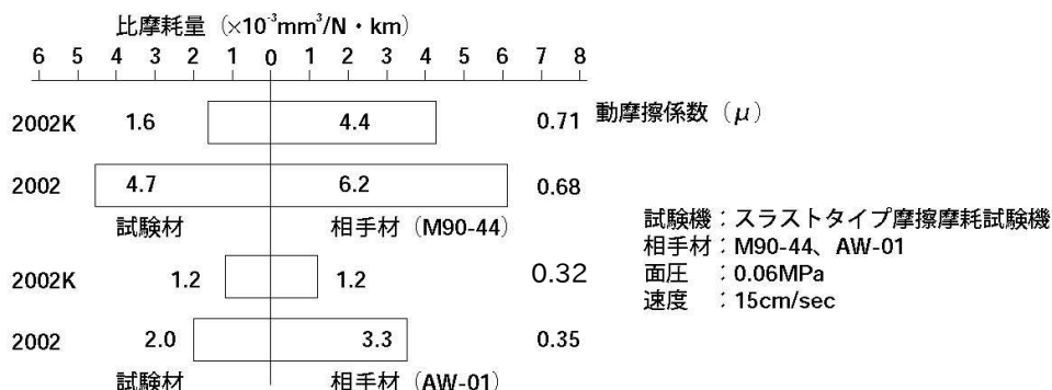
図2-1 対ジュラコンの摩擦摩耗系数
