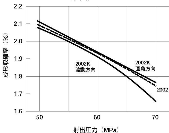
図2-3 成形収縮率 (120 \square \times 2mm \phi )
