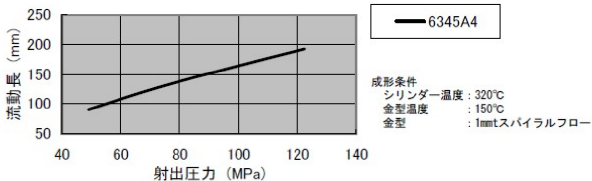
図 3-1 流動長(1mmt)
