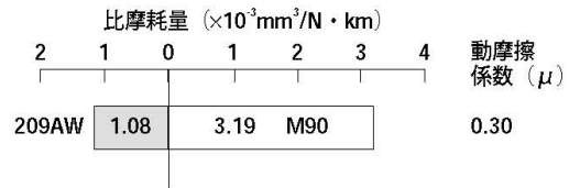
図3 対ジュラコンの摩擦磨耗系数
