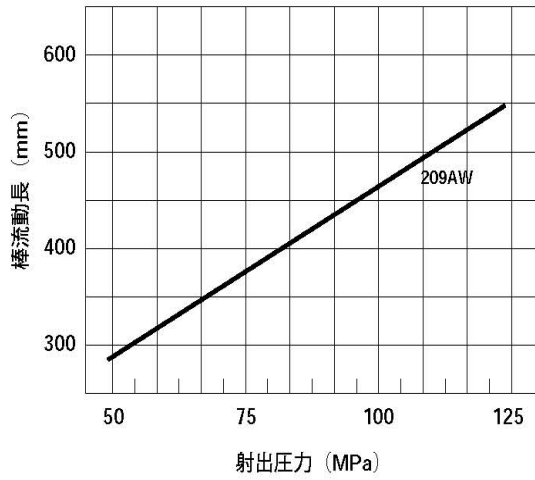
図4 棒流動長 (2mm \phi )
