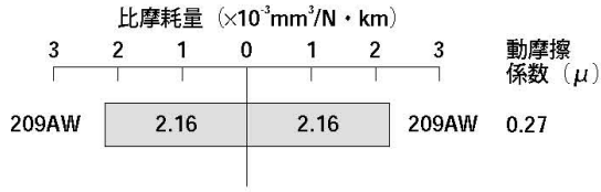
図1 対ジュラネックスの摩擦磨耗系数
