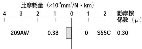
図2 対S55Cの摩擦磨耗系数
