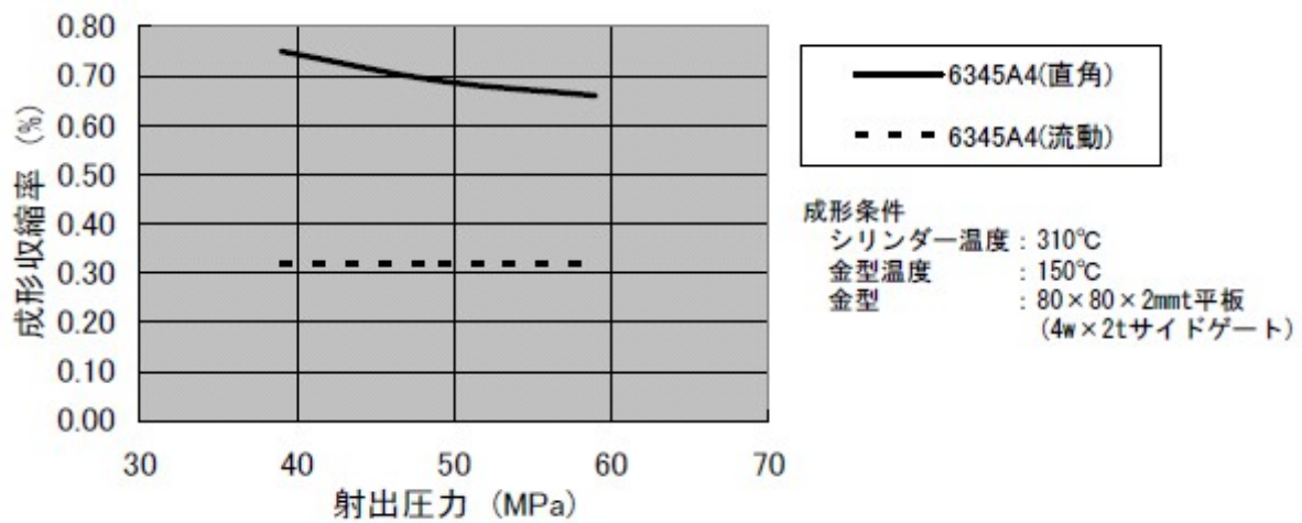
(図 3-2) 成形収縮率(80□×2mmt)
