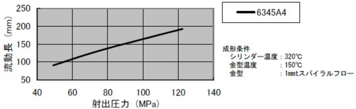
(図 3-1) 流動長(1mmt)
