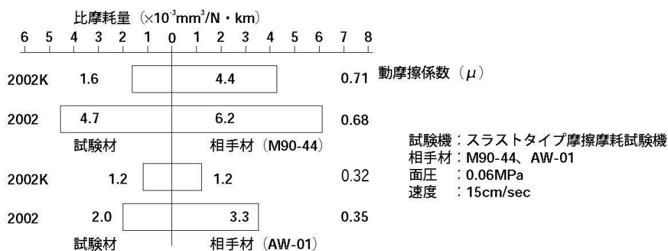
図2-1 対ジュラコンの摩擦摩耗系数
