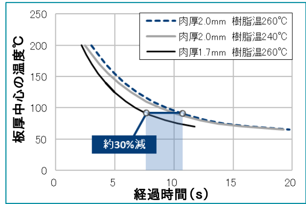
図2-3 薄肉化によるサイクル短縮
