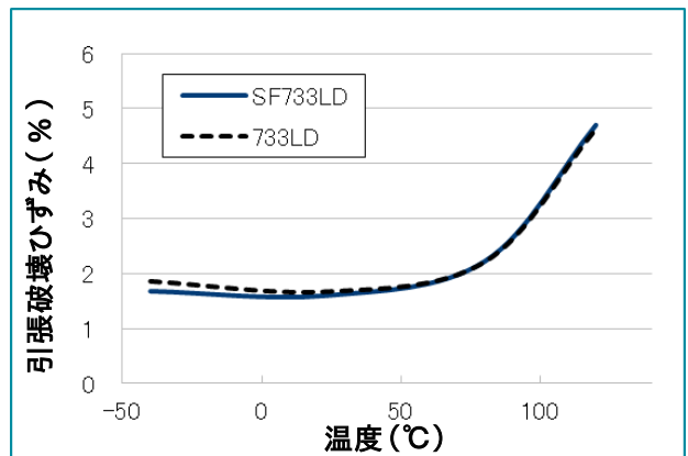
図6-2 温度依存性の比較(引張破壊ひずみ)
