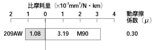
図3 対ジュラコンの摩擦磨耗係数
