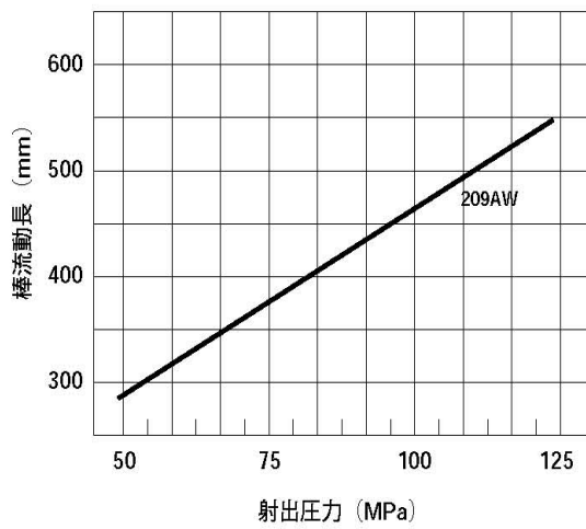
図4 棒流動長 (2mm t )
