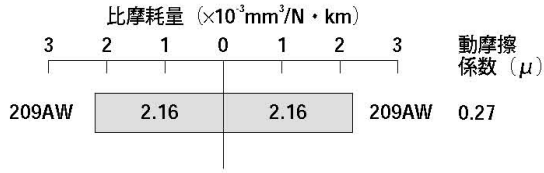
図1 対ジュラネックスの摩擦磨耗係数
