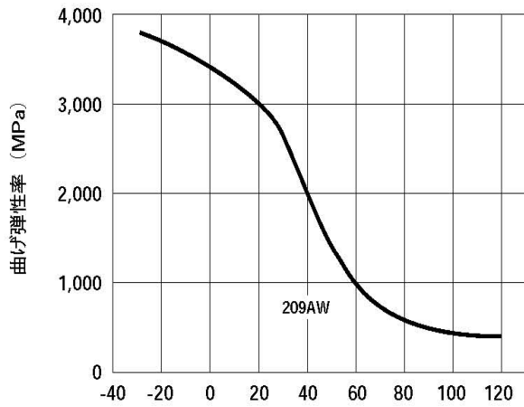
図7 曲げ弾性率の温度依存性
