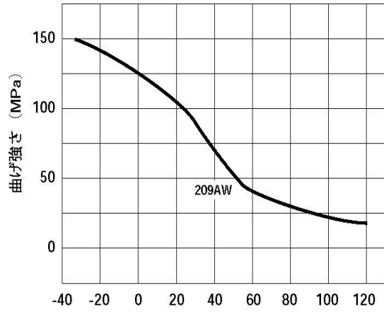
図6 曲げ強さの温度依存性
