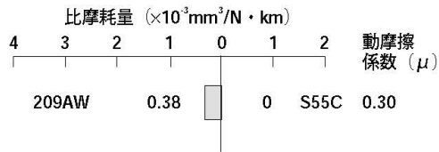
図2 対S55Cの摩擦磨耗係数
