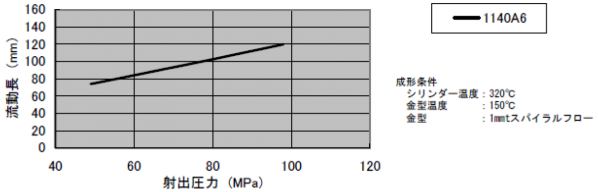
図 3-1 流動長(1mmt)
